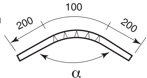
Colmo curvo sviluppo minimo 500 mm
