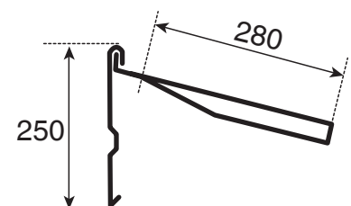
Colmo a shed stampato sviluppo minimo 625 mm
